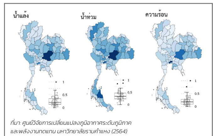
รูปที่ 11 ภัยและความเสี่ยงโดยรวมในสาขาการจัดการทรัพยากรน้ำ
