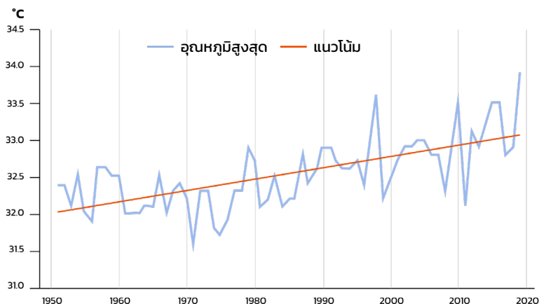
รูปที่ 7 แนวโน้มอุณหภูมิสูงสุดเฉลี่ยต่อปีของประเทศไทย
