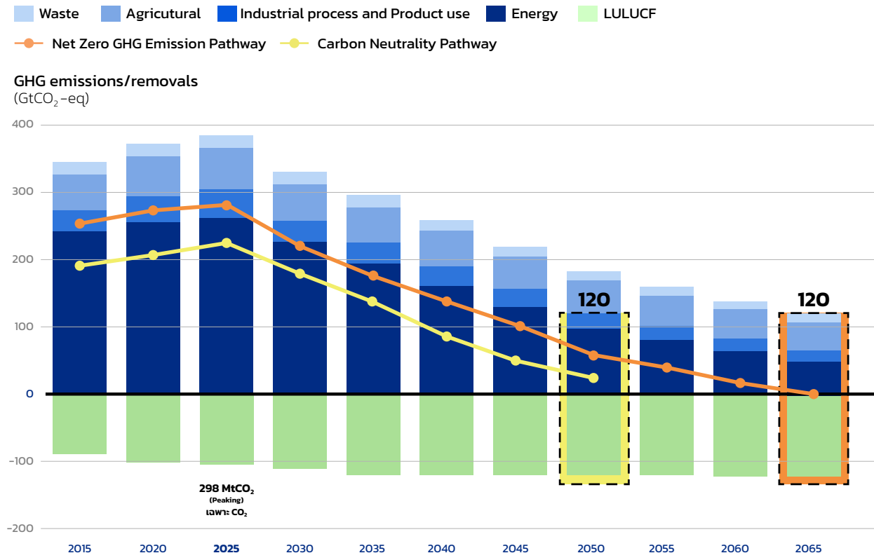
รูปที่ 21 ประมาณการปล่อยก๊าซเรือนกระจกในอนาคตของประเทศไทย แยกตามรายสาขา
