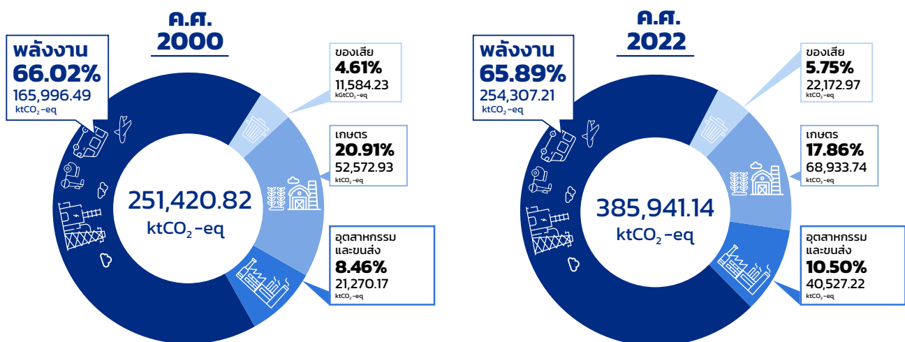
รูปที่ 20 เปรียบเทียบปริมาณการปล่อยก๊าซเรือนกระจกของไทย ปี พ.ศ. 2543 และ 2565
